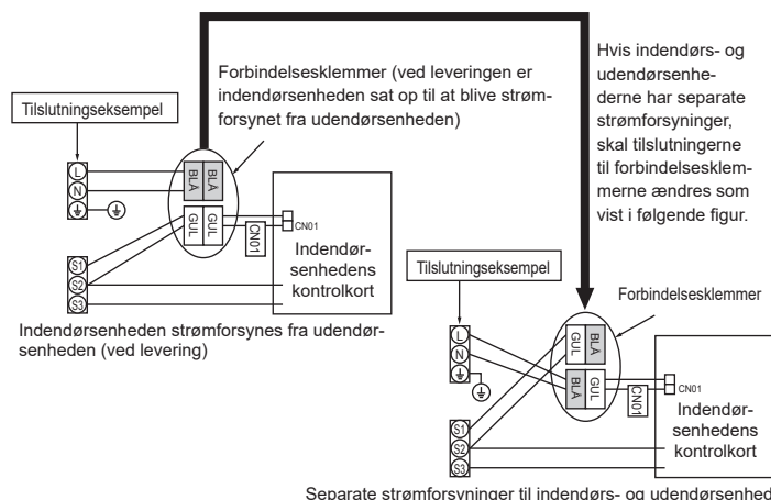
Separate strømforsyninger til indendørs- og udendørsenhed
