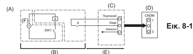
(Α) Παράδειγμα διαγράμματος κυκλώματος (Λειτουργία με χαμηλότερα επίπεδα θορύβου) (Β) Επιτόπου επέμβαση (C) Εξωτερικός διακόπτης δυαδικής εισαγωγής (PAC-SC36NA-E) (D) Πίνακας ελέγχου εξωτερικής μονάδας (Ε) Μέγ. 10 m (F) Παροχή ρεύματος για το ρελέ X: Ρελέ
