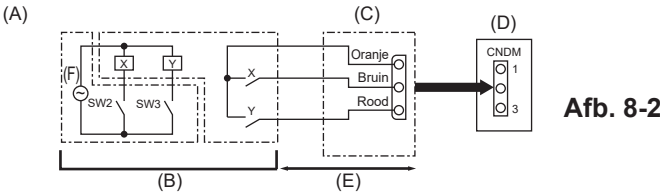
(A) Voorbeeld van elektrisch schema (Vraagfunctie) (C) Externe invoeradapter (PAC-SC36NA-E) (B) Indeling ter plaatse (D) Bedieningspaneel buitenapparaat X, Y: Relais (E) Max. 10 m (F) Stroomvoorziening voor relais
