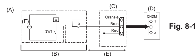
(A) Eksempel på koplingsskjema (lav støy-modus) (D) Utendørsenhets kontrollpanel (B) Ordnes på stedet (E) Maks. 10 m (C) Ekstern inngangsadapter (PAC-SC36NA-E) (F) Strømkilde for relé X: Relé
