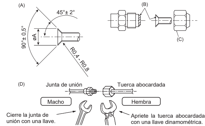
(A) Dimensiones del corte abocinado (D) Torsión de apriete de la tuerca abocardada
