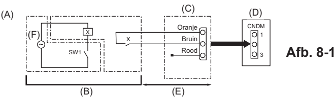
(A) Voorbeeld van elektrisch schema (stille werking) (D) Bedieningspaneel buitenapparaat (B) Indeling ter plaatse (E) Max. 10 m (C) Externe invoeradapter (PAC-SC36NA-E) (F) Stroomvoorziening voor relais X: Relais
