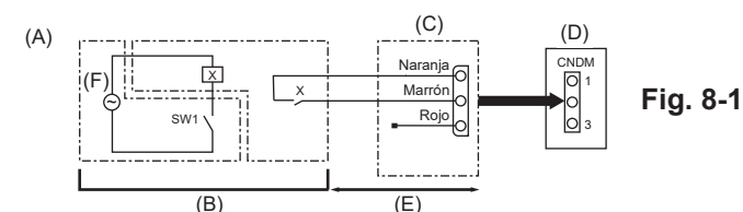
(A) Ejemplo de diagrama de circuito (modo de reducción del ruido) (B) Arreglo in situ (C) Adaptador de contacto externo (PAC-SC36NA-E) (D) Cuadro de control de la unidad exterior (E) Máx. 10 m (F) Fuente de alimentación del relé X: Relé
