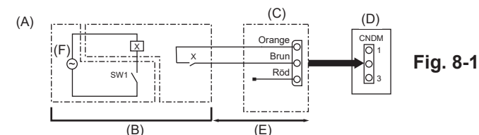
(A) Exempel på kopplingsschema (lägsta ljud-nivå) (B) Uppställning på plats (C) Yttre inadapter (PAC-SC36NA-E) X: Relä (D) Utomhusenhetens kontrollkort (E) Max. 10 m (F) Strömförsörjning för relä
