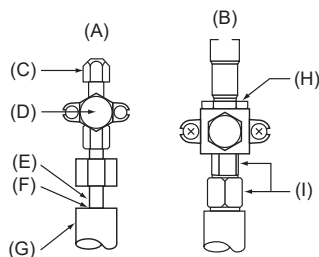
(A) Válvula <Lado do líquido> (B) Válvula <Lado do gás> (C) Porta de manutenção (D) Secção Abrir/Fechar (E) Tubo local (F) Vedado, tal como para o lado do gás (G) Cobertura do tubo (H) Não use a chave aqui. Pode provocar fuga de refrigerante. (I) Use aqui duas chaves.
