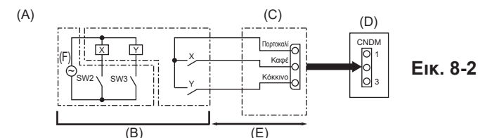
(Α) Παράδειγμα διαγράμματος κυκλώματος (Λειτουργία ρύθμισης) (Β) Επιτόπου επέμβαση (C) Εξωτερικός διακόπτης δυαδικής εισαγωγής (PAC-SC36NA-E) (D) Πίνακας ελέγχου εξωτερικής μονάδας (Ε) Μέγ. 10 m (F) Παροχή ρεύματος για το ρελέ X, Y: Ρελέ
