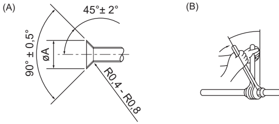
(A) Afsnijmaten tromp (B) Aanhaalmoment flensmoer
