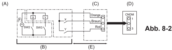
(A) Beispiel eines Schaltplans (Anforderungsfunktion) (C) Externer Eingangsadapter (PAC-SC36NA-E) (B) Anordnung vor Ort (D) Schalttafel der Außenanlage X, Y: Relais (E) Max. 10 m (F) Stromversorgung für Relais
