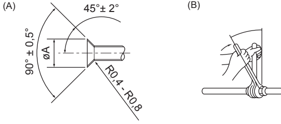
(A) Geçme kesim ölçüleri (B) Geçme somun sıkıştırma torku
