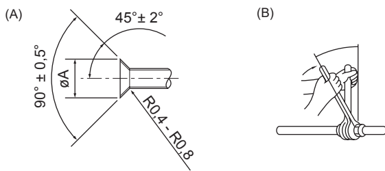
(A) Wymiary przycinania kielichów (B) Moment dokręcania nakrętek kielichowych
