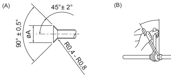
(A) Skæremål for kraver (B) Tilspændingsmoment for omløbermøtrik
