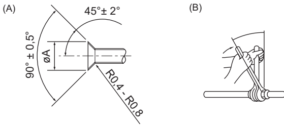
(A) Διαστάσεις εκχειλωσης (B) Ροπή σύσφιξης για το περικόχλιο εκχειλωσης
