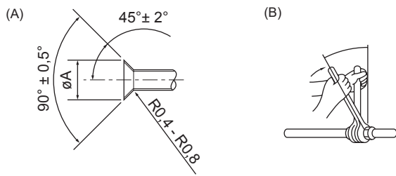
(A) Dimension de l'évasement (B) Couple de serrage du raccord conique
