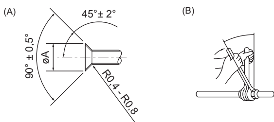
(A) Mått för flänsning (B) Åtdragningsmoment för flänsmutter
