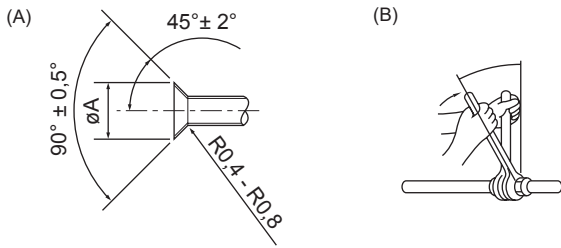
(A) Dimensioni di taglio per raccordo a cartella (B) Coppia di serraggio del dado a cartella
