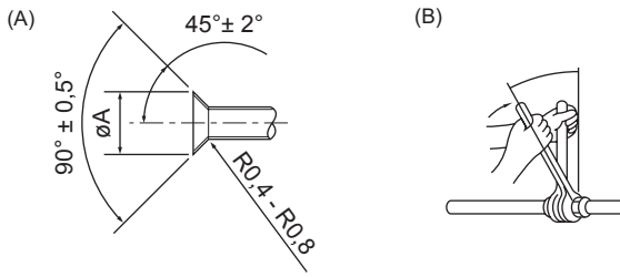
(A) Abmessungen der Aufweitungsschnitte (B) Anzugsdrehmoment für die Konusmutter
