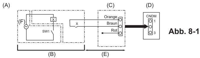
(A) Beispiel eines Schaltplans (Lärmschutzmodus) (D) Schalttafel der Außenanlage (B) Anordnung vor Ort (E) Max. 10 m (C) Externer Eingangsadapter (PAC-SC36NA-E) (F) Stromversorgung für Relais X: Relais
