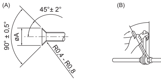
(A) Dimensões do corte de afunilamento (B) Binário de aperto da porca afunilada
