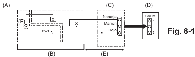
(A) Ejemplo de diagrama de circuito (modo de reducción del ruido) (B) Arreglo in situ (C) Adaptador de contacto externo (PAC-SC36NA-E) X: Relé (D) Cuadro de control de la unidad exterior (E) Máx. 10 m (F) Fuente de alimentación del relé
