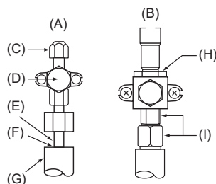
(A) Vanne <côté liquide> (B) Vanne <côté gaz> (C) Orifice pour l'entretien (D) Section d'ouverture/fermeture (E) Tuyau local (F) Hermétique, idem pour le côté gaz (G) Fourrure du tuyau (H) Ne pas utiliser de clé ici. Il pourrait y avoir des fuites de réfrigérant. (I) Utiliser deux clés ici.
