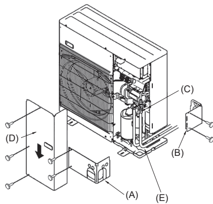
(A) Vordere Leitungsabdeckung (B) Leitungsabdeckung (C) Ventil (D) Wartungspult (E) Radius der Biegung : 100 mm - 150 mm
