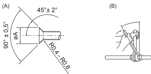
(A) Wymiary przycinania kielichów (B) Moment dokręcania nakrętek kielichowych
