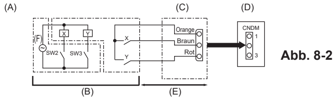
(A) Beispiel eines Schaltplans (Anforderungsfunktion) (C) Externer Eingangsadapter (PAC-SC36NA-E) (B) Anordnung vor Ort (D) Schalttafel der Außenanlage X, Y: Relais (E) Max. 10 m (F) Stromversorgung für Relais
