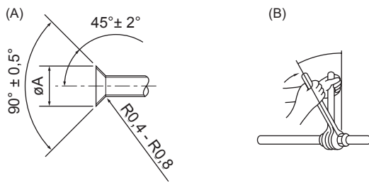
(A) Leppeskjæringsdimensjoner (B) Tiltrekkingsmoment for leppemutter
