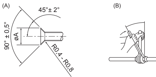
(A) Mått för flänsning (B) Åtdragningsmoment för flänsmutter
