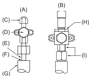
(A) Válvula <Lado do líquido> (B) Válvula <Lado do gás> (C) Porta de manutenção (D) Secção Abrir/Fechar (E) Tubo local (F) Vedado, tal como para o lado do gás (G) Cobertura do tubo (H) Não use a chave aqui. Pode provocar fuga de refrigerante. (I) Use aqui duas chaves.
