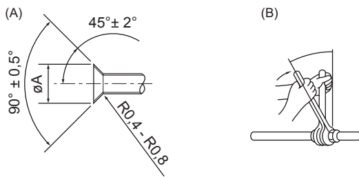
(A) Skæremål for kraver (B) Tilspændingsmoment for omløbermøtrik
