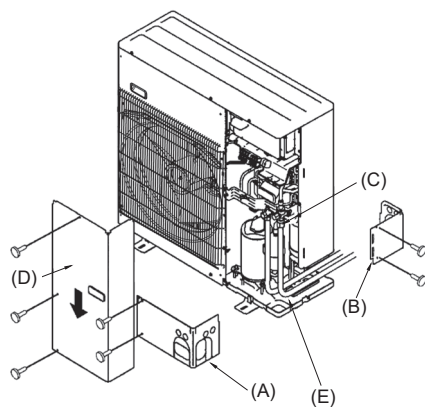
(A) Frontdæksel til rørføring (B) Rørføringsdæksel (C) Ventil (D) Servicepanel (E) Bøjeradius : 100 mm - 150 mm
