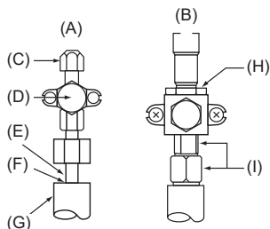
(A) Ventil <Flüssigkeitsseite> (B) Ventil <Gasseite> (C) Ausgang der Wartungseinheit (D) Abschnitt öffnen/schließen (E) Hausrohrleitung (F) Versiegelt wie auf der Gasseite (G) Rohrabdeckung (H) Hier keinen Schraubenschlüssel verwenden. Es kann Austritt von Kältemittel zur Folge haben. (I) Hier zwei Schraubenschlüssel verwenden.
