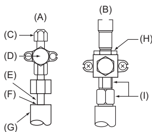
(A) Valve <Liquid side> (B) Valve <Gas side> (C) Service port (D) Open/Close section (E) Local pipe
