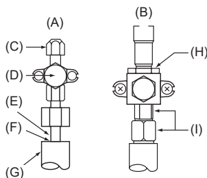
(A) Válvula <Lado de líquido> (B) Válvula <Lado de gas> (C) Puerto de servicio (D) Sección Abierto/Cerrado (E) Tubo local
