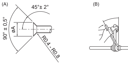
(A) Διαστάσεις εκχειλωσης (B) Ροπή σύσφιξης για το περικόχλιο εκχειλωσης
