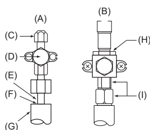
(A) Ventil <væskeside> (B) Ventil <gasside> (C) Serviceport (D) Åbne/lukke-sektion (E) Pladsmonteret rør
