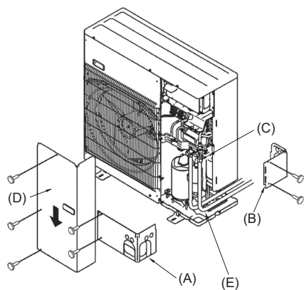
(A) Cubierta de la tubería frontal (B) Cubierta de la tubería posterior (C) Válvula (D) Panel de servicio (E) Radio del codo: 100 mm-150 mm
