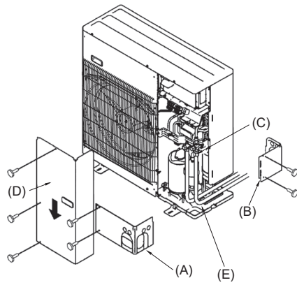
(A) Coperchio della tubazione anteriore (B) Coperchio del tubo (C) Valvola (D) Pannello di servizio (E) Raggio della curva : 100 mm - 150 mm
