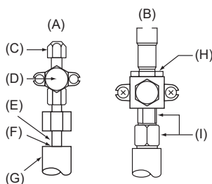
(A) Ventil <vätskesida> (B) Ventil <gassida> (C) Serviceöppning (D) Öppen/stängd sektion (E) Lokalt rör (F) Tätad, på samma sätt som på gassidan (G) Rörskydd (H) Använd inte skruvnyckel här. Kylmedelsläckage kan uppstå. (I) Använd två skruvnycklar här.
