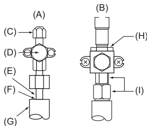
(A) Valvola <Lato liquido> (B) Valvola <Lato gas> (C) Attacco di servizio (D) Sezione Aperto/Chiuso (E) Tubazione locale (F) Sigillato, come per il lato gas (G) Coperchio del tubo (H) Non utilizzare una chiave in questo punto. Possono verificarsi perdite di refrigerante. (I) Utilizzare due chiavi in questo punto.
