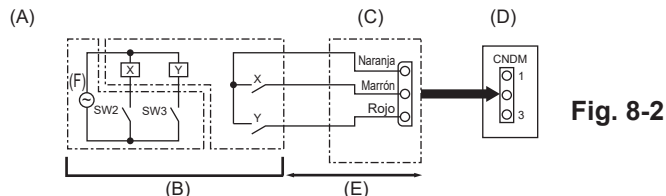
(A) Ejemplo de diagrama de circuito (Función de demanda) (B) Arreglo in situ X, Y: Relé (C) Adaptador de contacto externo (PAC-SC36NA-E) (D) Cuadro de control de la unidad exterior (E) Máx. 10 m (F) Fuente de alimentación del relé
