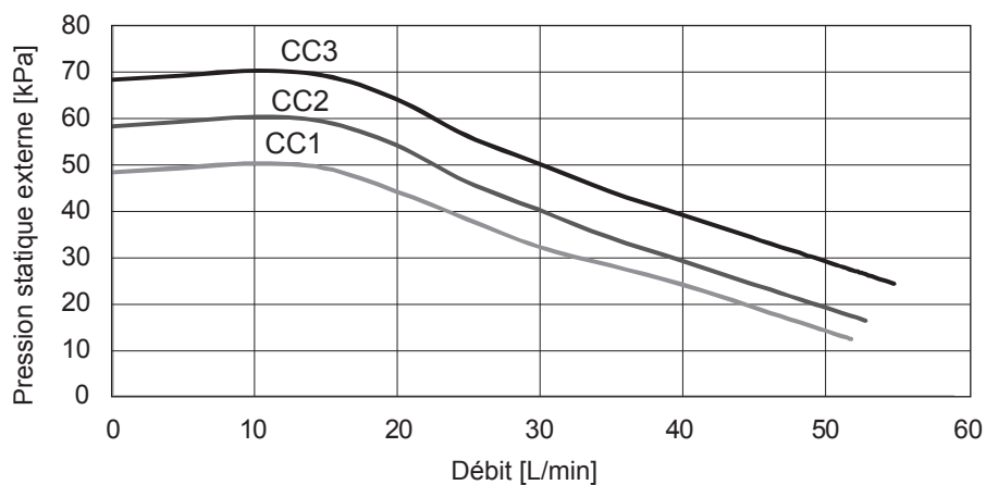
<Courbe Constante>
