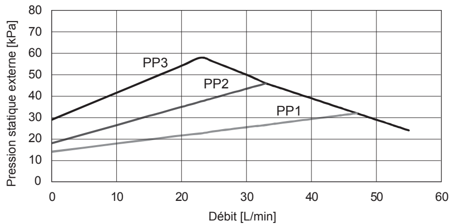
<Pression Proportionnelle>
