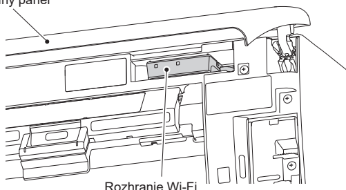
Rozhranie Wi-Fi
