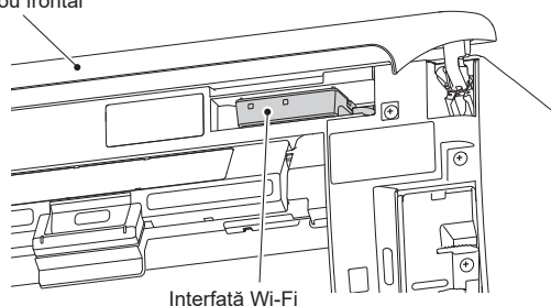
Interfață Wi-Fi
