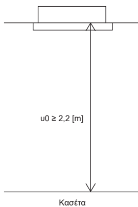
Κασέτα
