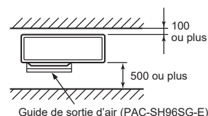
Guide de sortie d'air (PAC-SH96SG-E)
