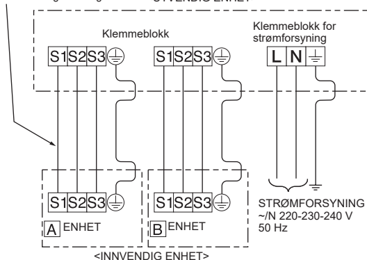
Koblingsledning mellom innvendig/utvendig enhet <UTVENDIG ENHET>
