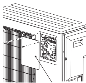
Panel serwisowy
