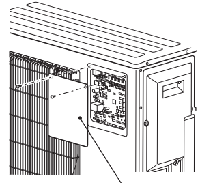
Bakım paneli
