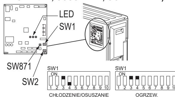
Panel serwisowy
