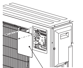
Panneau d'entretien
