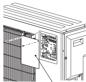
Panel serwisowy
