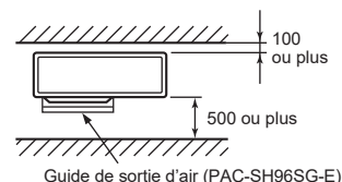
Guide de sortie d'air (PAC-SH96SG-E)
