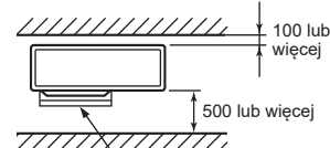
Kierownica wylotowa powietrza (PAC-SH96SG-E)
