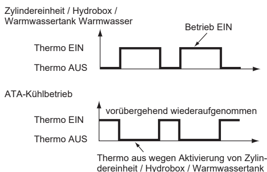
Betriebszustand bei gleichzeitiger Anforderung von ATA-Kühlbetrieb und Warmwasserbereitung
