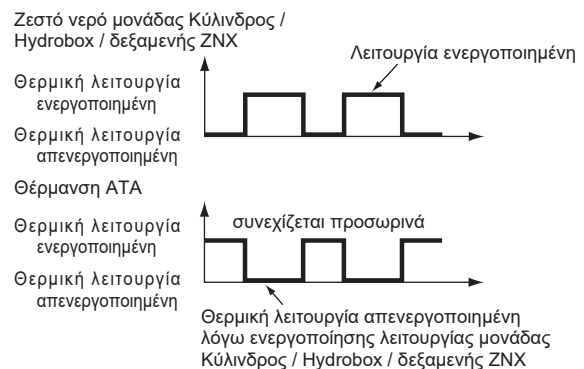
Κατάσταση λειτουργίας όταν ζητούνται ταυτόχρονα οι λειτουργίες θέρμανσης ATA και παροχής ζεστού νερού
