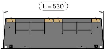
BTT - Bac 2 travées 13 modules
