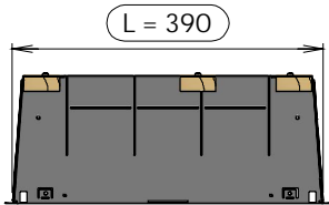
BTM - Bac 1 travée 18 modules
