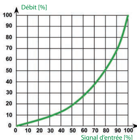
AB-QM + AME 435 QM avec réglage sur logarithmique
