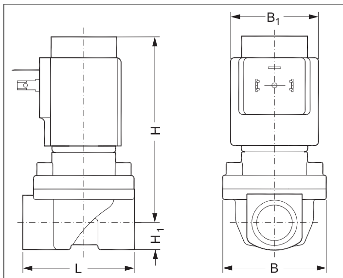
Chiffre 4: Dimensions
