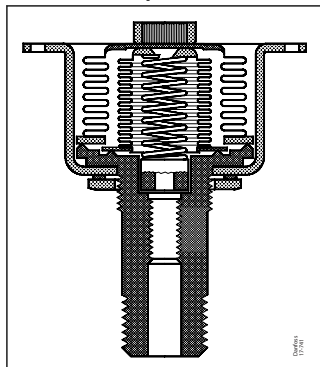
Chiffre 5: Coupe transversale du RT 30W
