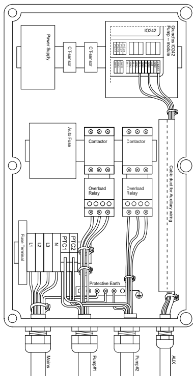
Connexions triphasées pour deux pompes
