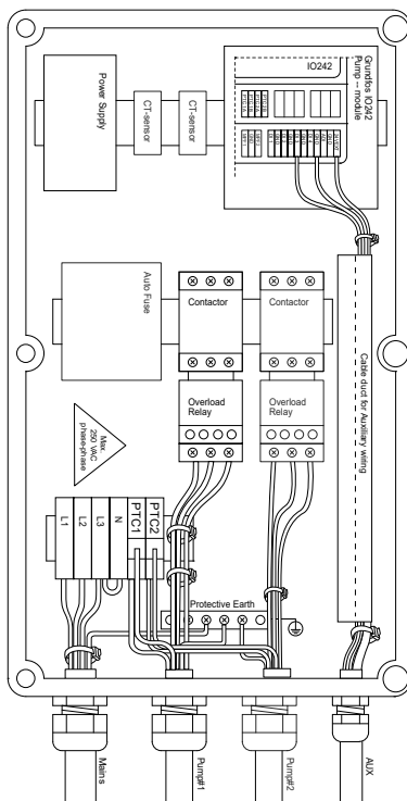
Connexions triphasées pour deux pompes sans neutre (Norvège uniquement)
