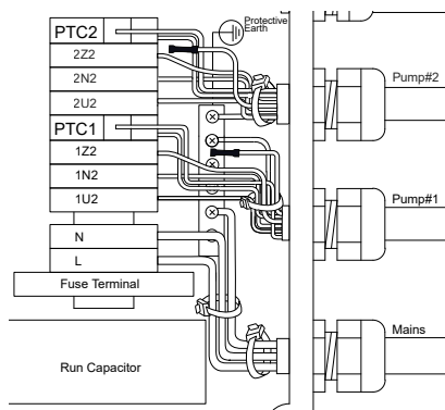
Câblage PTC recommandé
