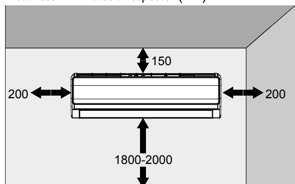
Distances minimales à respecter (mm)
