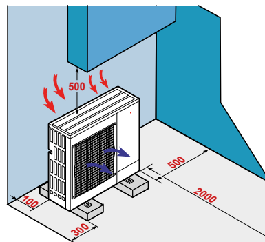
Distances minimales à respecter (mm)
