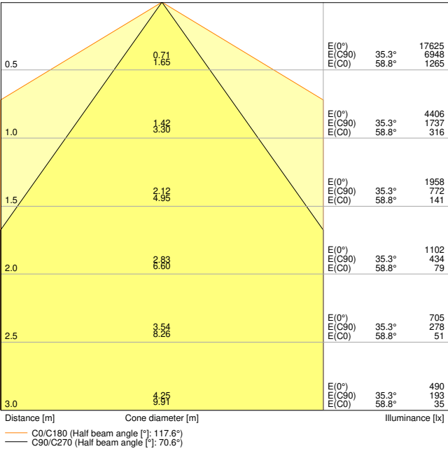
TRUSYS FLEX P 70W 840 DS CL WT DALI
