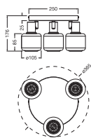
DECOR SPOT FIREFLY PL 3X2.8W E14 BK
