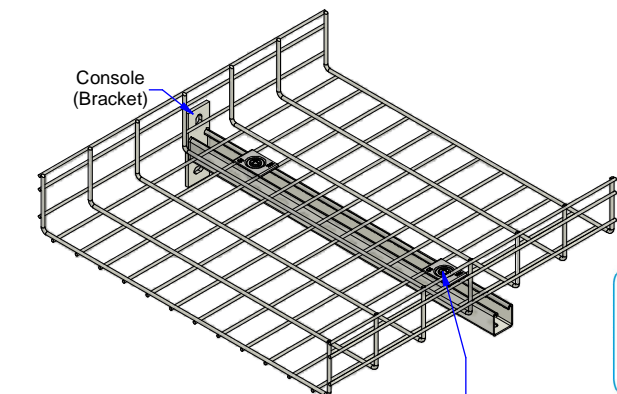
BP TRL + Ecrou rainuré M6 (BP TRL + Nut M6 Strut)
