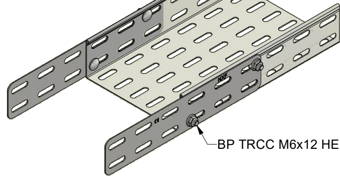
Goulotte GBRs (GBRS Trunking)
