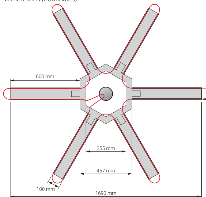
Dimensions (nominales)
