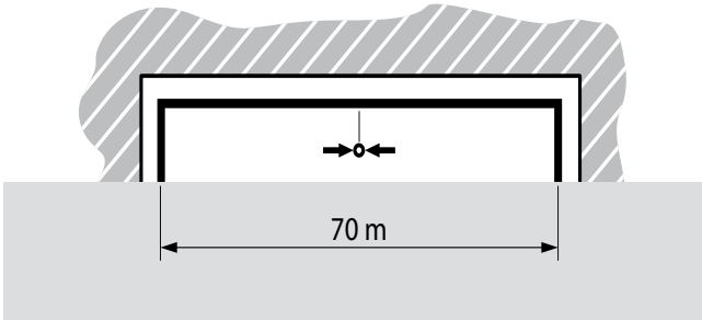
Longueur de la section droite 70 m = 1 élément de dilatation au centre
