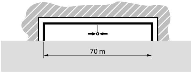
Longueur de la section droite 70 m = 1 élément de dilatation au centre
