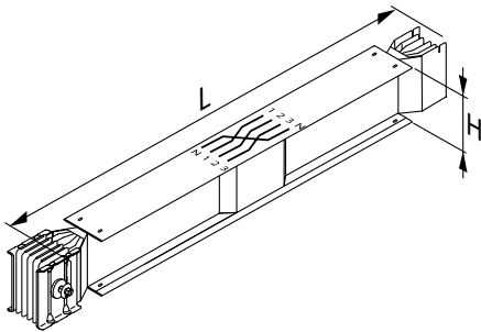
Dimensions : L 1000 mm x H 440 mm
