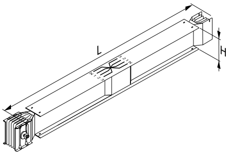
Dimensions : L 1200 mm x H 440 mm
