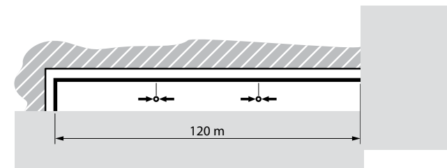
Longueur de la section droite 120 m = 2 éléments de dilatation soit 1 tous les 40 m
