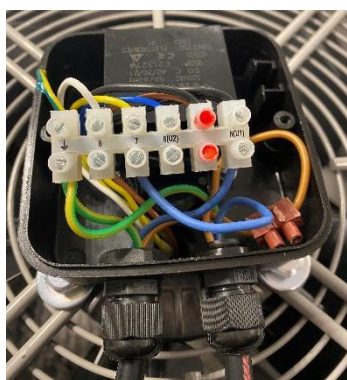
Bornier déstratificateur DS6500
