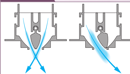
Déflecteur en position médiane ou complètement ouvert.
