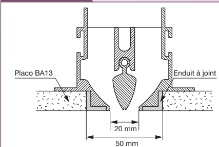
Vu en coupe de l'installation sur placo.
