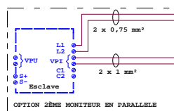
PLATINE SECONDAIRE PLAQUE DE RUE VIDEO
