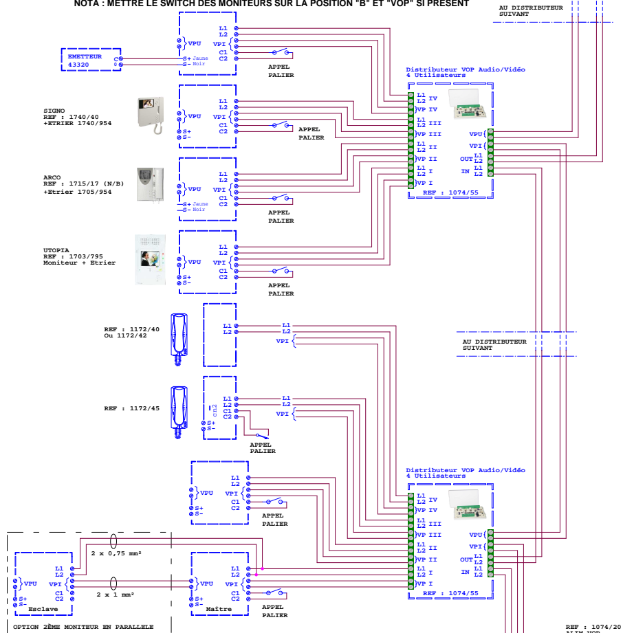
PLATINE SECONDAIRE PLAQUE DE RUE VIDEO
