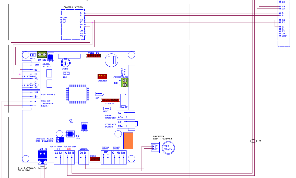
PLATINE SECONDAIRE PLAQUE DE RUE VIDEO
