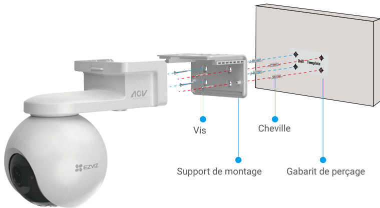
Fig. 2 Montage mural
