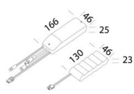
600 Kit d'alimentation SEC.
