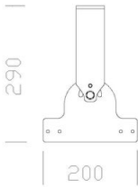
530 Étrier orientable
