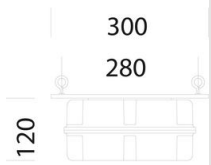
1175 Boîtier SEC. - 997654-00
