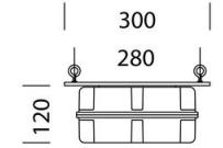
1175 Boîtier SEC. - 997651-00
