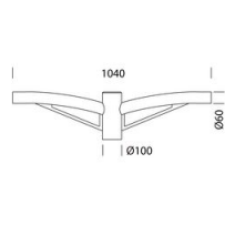
508 Bras double
