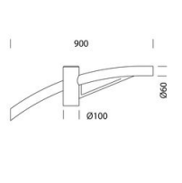
504 Bras simple
