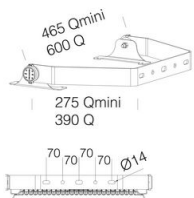
38 étrier mural
