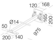
42 Bras orientable
