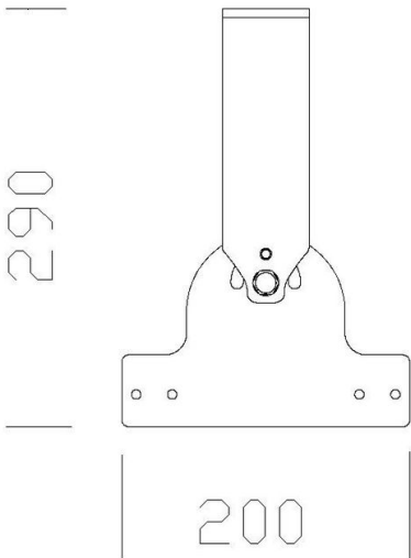
530 Staffa orientabile
