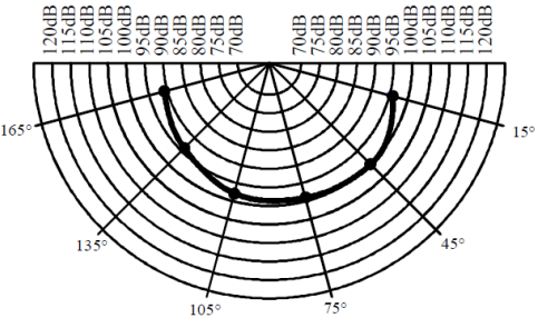
Diagramme Polaire de la tonalité 11
