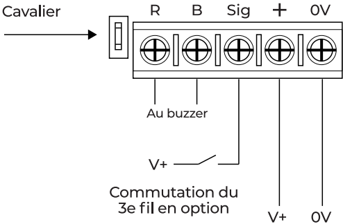
Schéma câblage 1 (Vcc)
