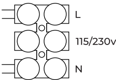
Schéma câblage 4 (Vca)
