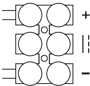
Schéma câblage 3 (Vca/cc)
