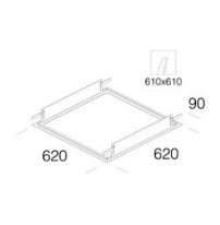
Cadre - 620x620
