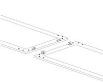
Étriers d'alignement
