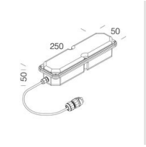
Boîtier d'alimentation IP65 pour version standard 500 mA
