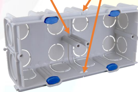
Les boîtiers s'emboîtent à l'aide des glissières en partie haute et basse, et se verrouillent en partie arrière.
