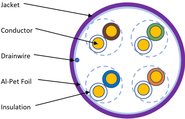
Dessin de la section du câble
