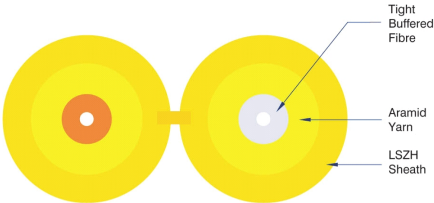
Dessin de la section du câble
