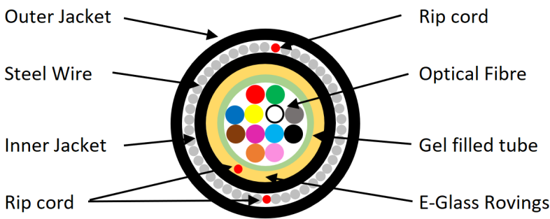
Dessin de la section du câble
