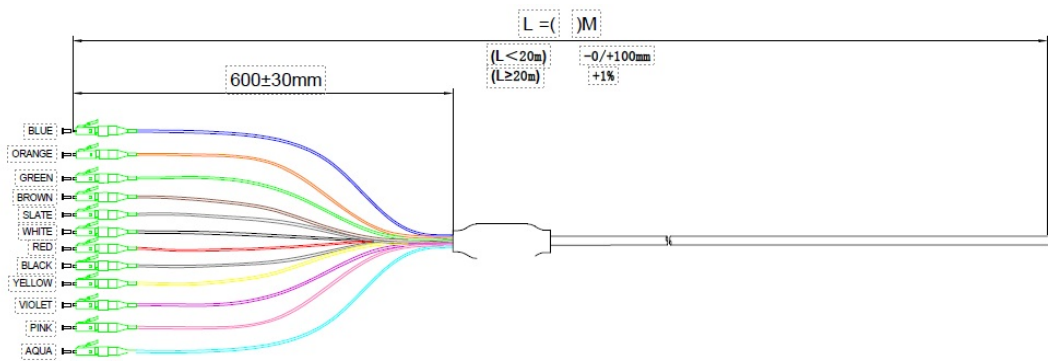
Dessin de la section du câble
