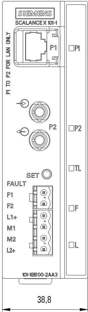
Vorne / Front
